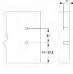
dimensões de perfuração do painel frontal
