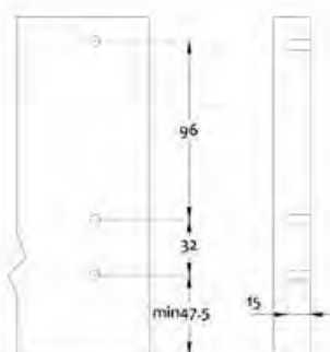
dimensões de perfuração do painel frontal
