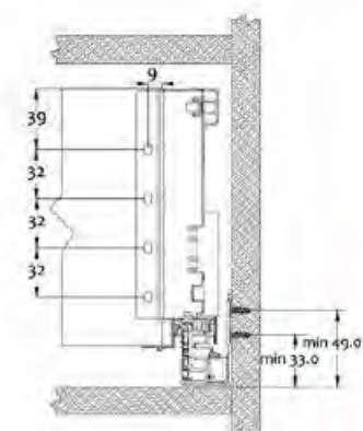
dimensões de instalação do painel traseiro
