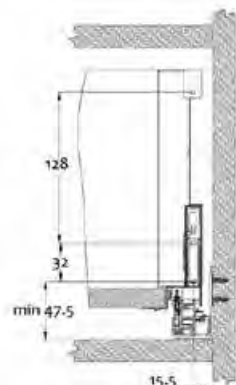
dimensões de instalação do painel do conector frontal
