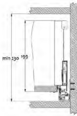
espaço necessário no armário
