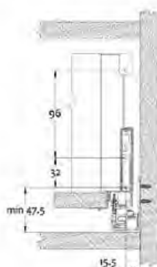
dimensões de instalação do painel do conector frontal
