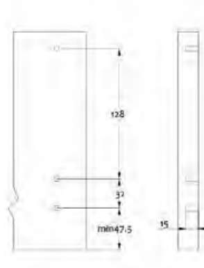
dimensões de perfuração do painel frontal
